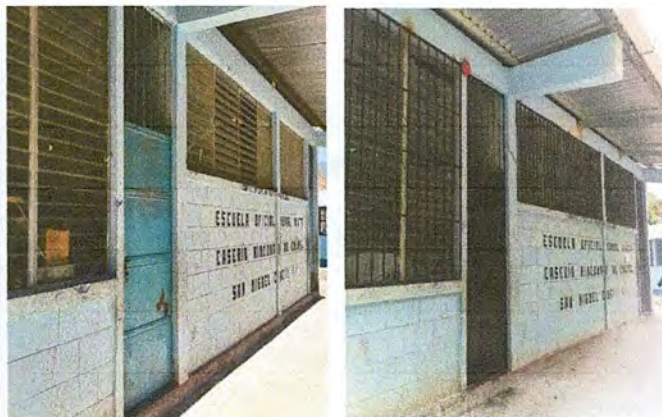
Foto 2: MEJORAMIENTO E INSTALACION DE BALCONES
